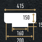
DC-8303C-8H (150x415x140 мм)
