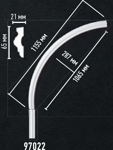
897022-150 (R нар. - 815 мм, R вн. - 750 мм)
