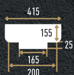
DC-8303C-8 (155x415x280 мм)
