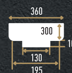
90018-1H (300x360x180 мм)
