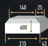
DK-202 (600x215x43 мм)
