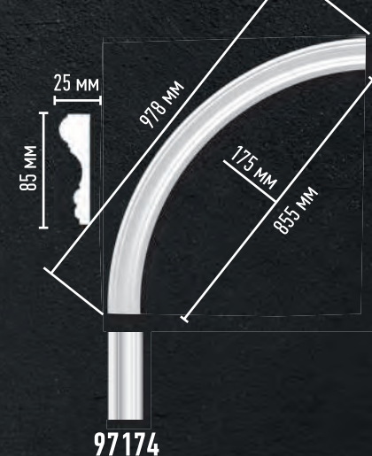
897174-120 (R нар. - 685 мм, R вн. - 600 мм)
