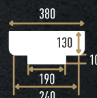
90024-3 (130xØ380 мм)
