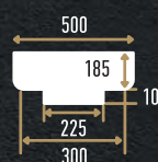
90030-2H (185x500x250 мм)
