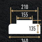
DCK-21H (135xØ340x170 мм)
