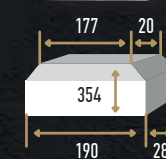
DK-82222 (354x190x28 мм)
