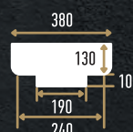
90024-3 (130xØ380 мм)
