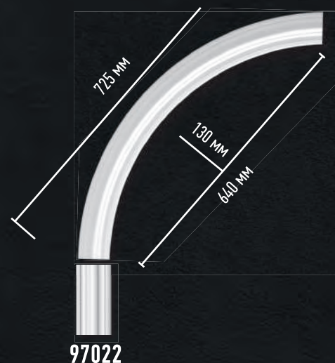
897022-90 (R нар. - 515 мм, R вн. - 450 мм)
