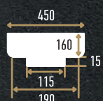
90024-2 (160x450x450 мм)
