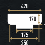
90024-5 (170x420x420 мм)
