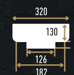
90018-3H (130x320x155 мм)
