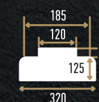
90018-4 (125xØ320 мм)
