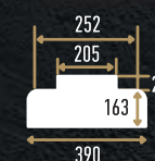
DC-8302-8H (163xØ390x195 мм)
