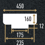
90024-2 (160x450x450 мм)
