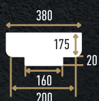
DCK-12 (175x380x380мм)
