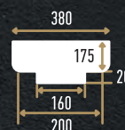
DCK-12 (175x380x380мм)
