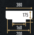
DCK-12 (175x380x380 мм)
