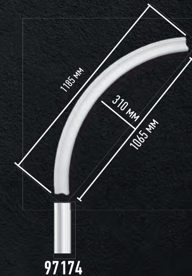
897174-150 (R нар. - 835 мм, R вн. - 750 мм)
