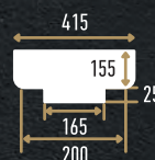
DC-8303C-8 (155x415x280 мм)
