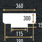
90018-1 (300x360x360 мм)
