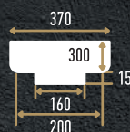
DCK-11H (300x370x185 мм)
