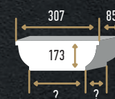
DK-82221 (173x307x85 мм)
