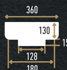
90018-2 (130x360x360 мм)
