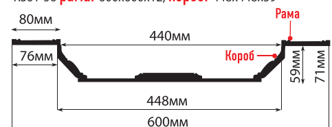
КС61-56 рама: 600x600x12, короб: 448x448x59
