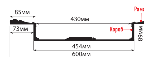
KS61A-19D рама: 600x600x25, короб: 454x454x89
