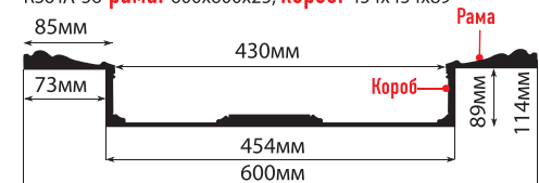
КС61А-56 рама: 600x600x25, короб: 454x454x89
