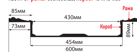
KS61A-57 рама: 600x600x25, короб: 454x454x89
